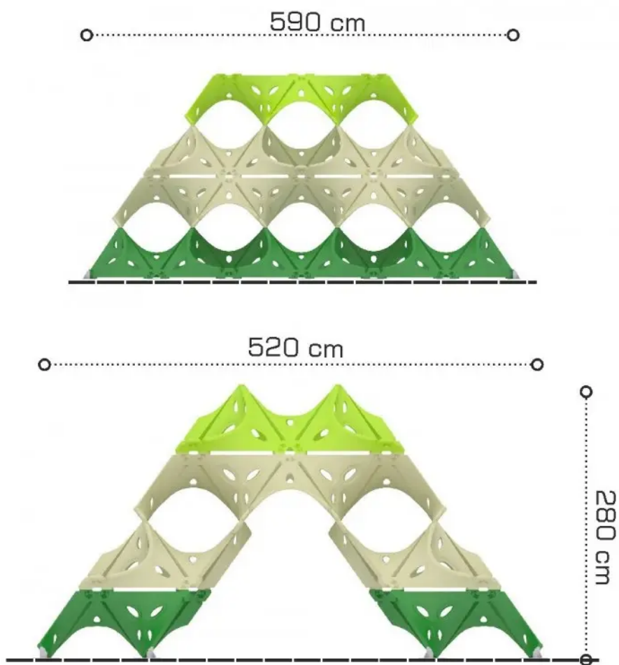
Rys. 1. Wymiary urządzenia
