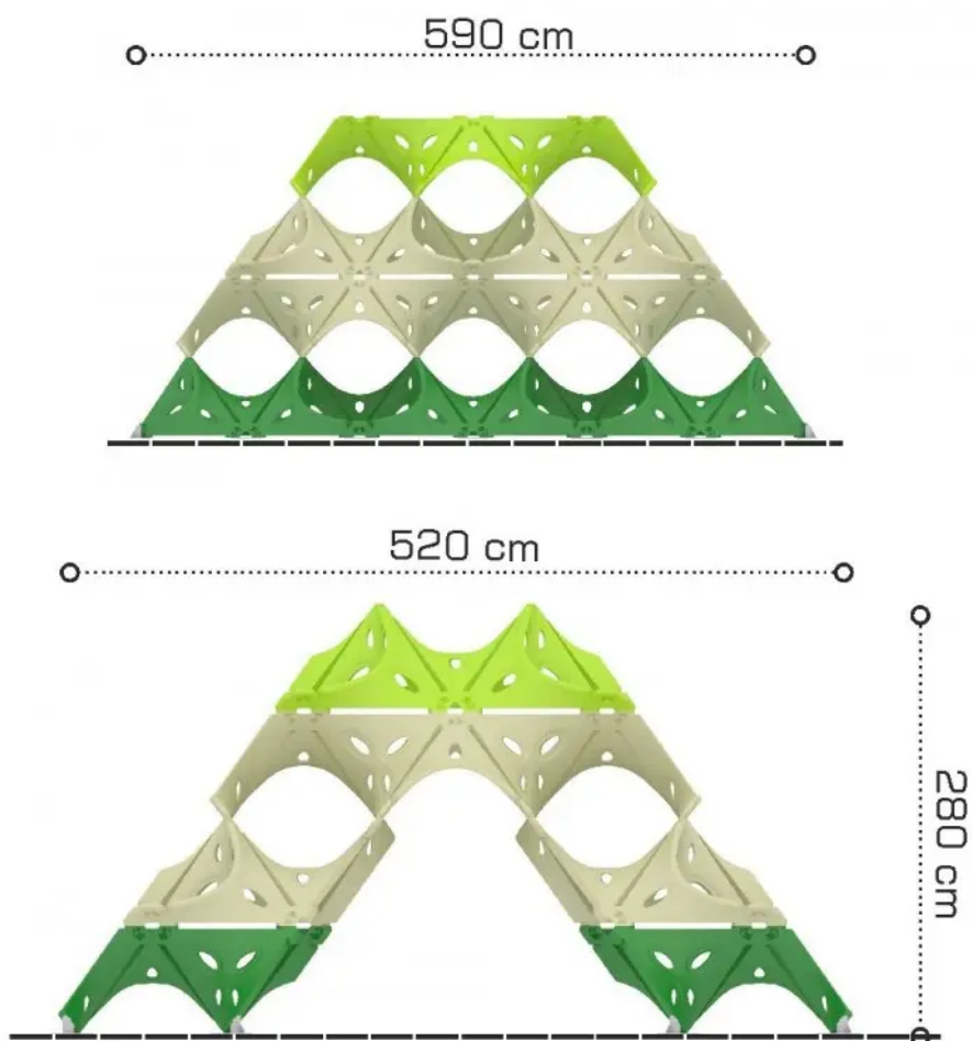
Rys. 1. Wymiary urządzenia
