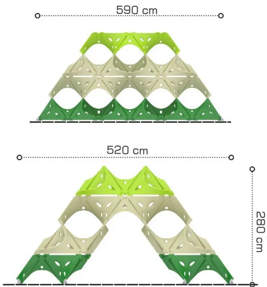
Rys. 1. Wymiary urządzenia
