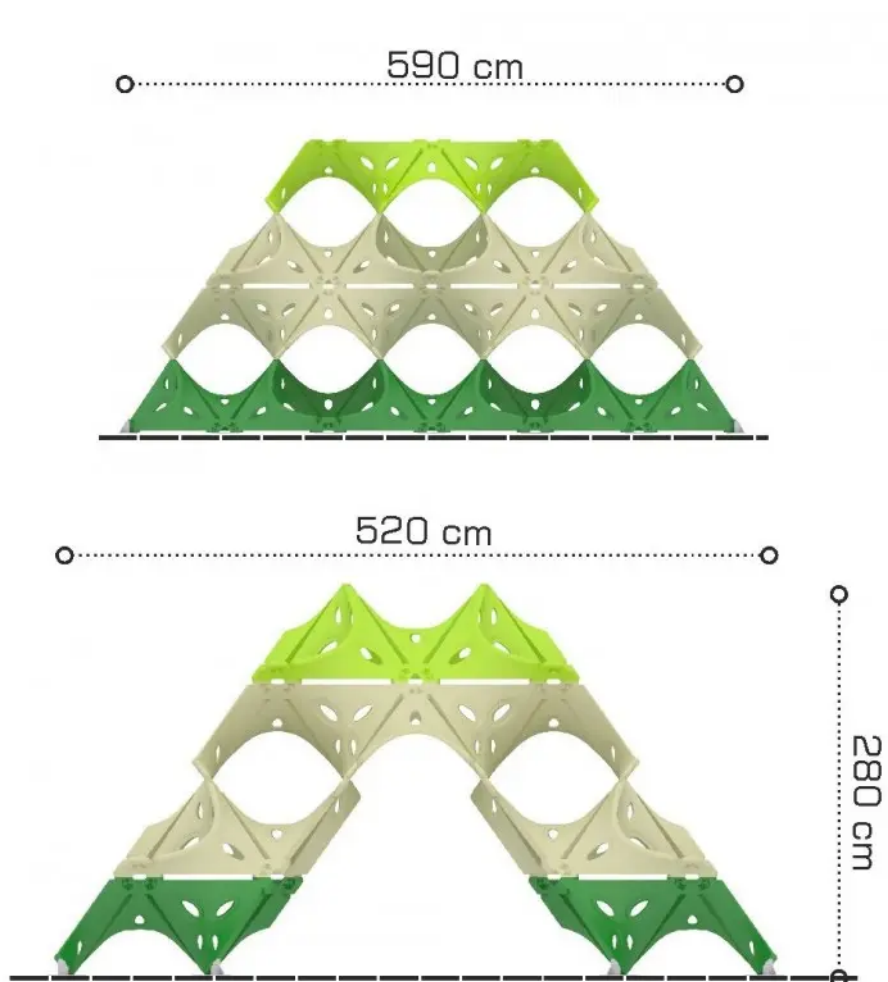
Rys. 1. Wymiary urządzenia
