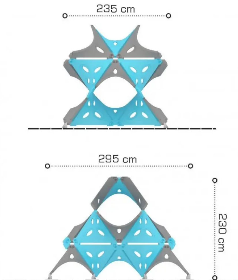
Rys. 1. Wymiary urządzenia
