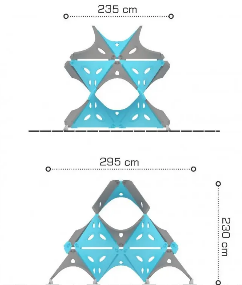
Rys. 1. Wymiary urządzenia
