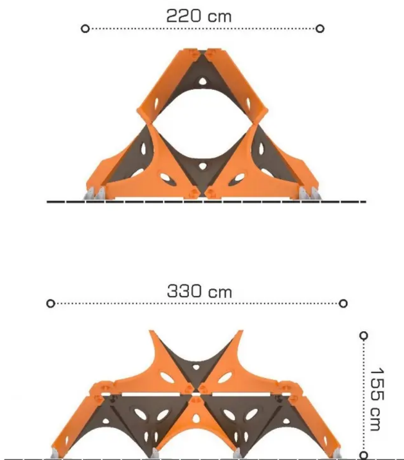
Rys. 1. Wymiary urządzenia
