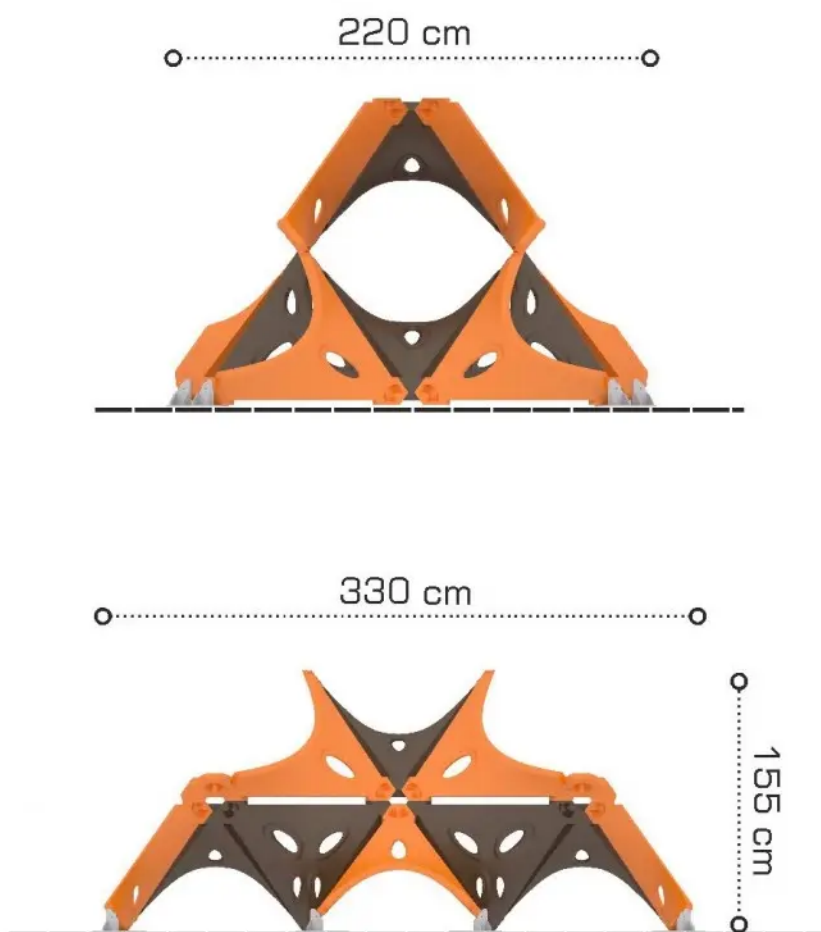
Rys. 1. Wymiary urządzenia
