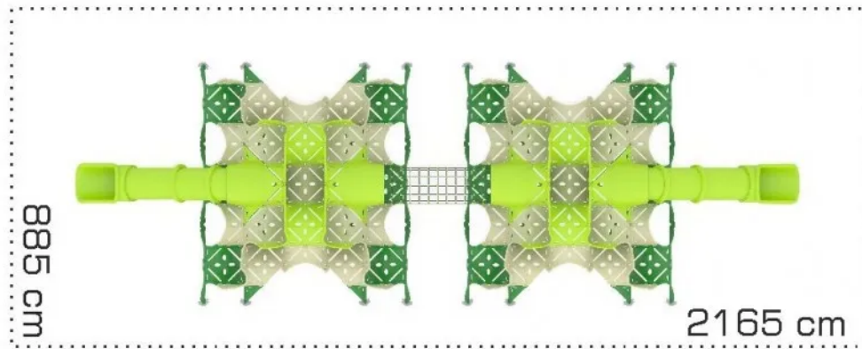
Rys. 2. Wymiary strefy bezpieczeństwa
