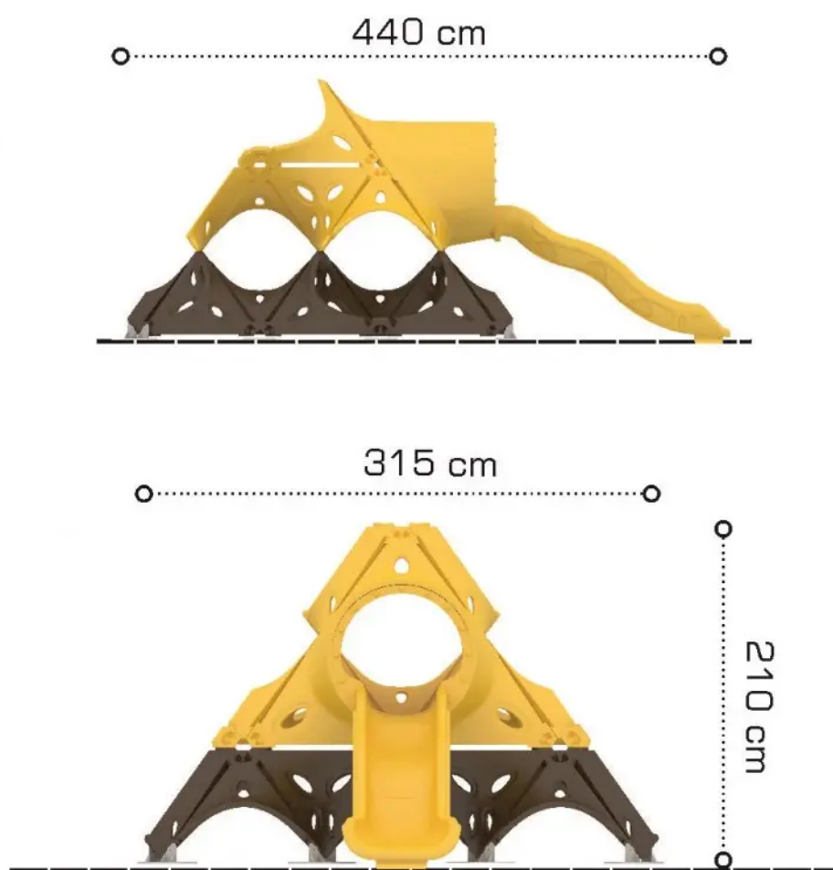
Rys. 1. Wymiary urządzenia
