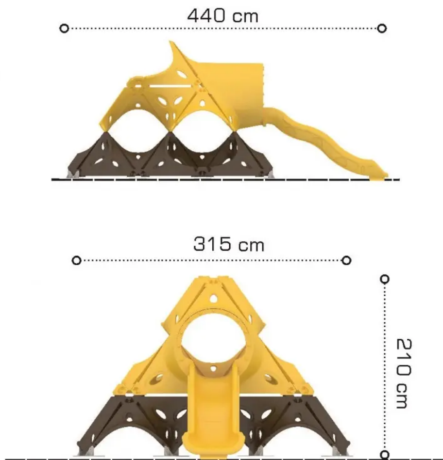
Rys. 1. Wymiary urządzenia
