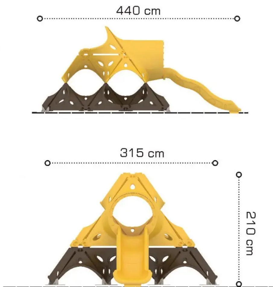
Rys. 1. Wymiary urządzenia
