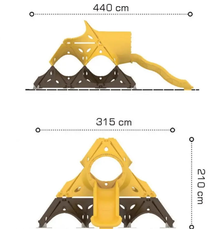
Rys. 1. Wymiary urządzenia
