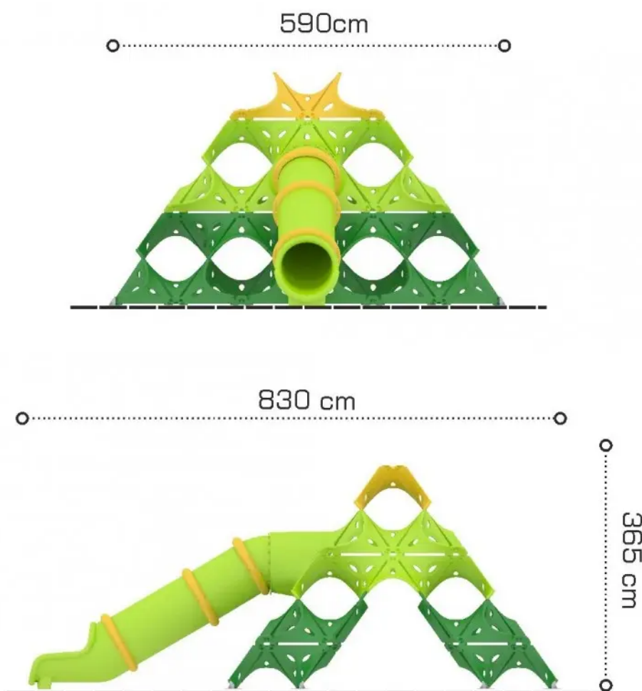
Rys. 1. Wymiary urządzenia
