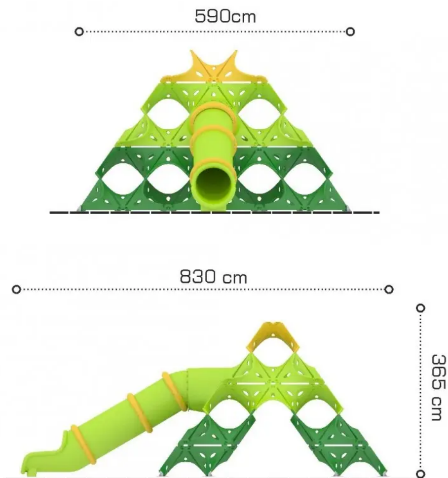
Rys. 1. Wymiary urządzenia
