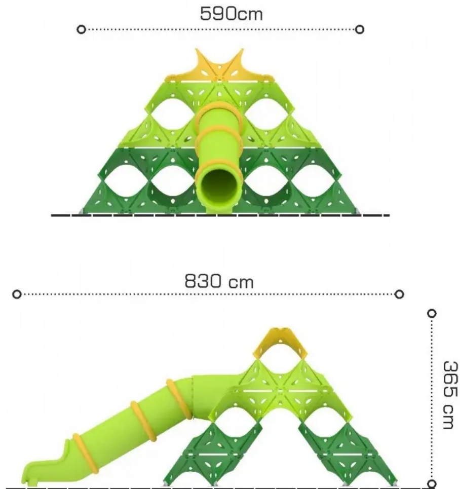
Rys. 1. Wymiary urządzenia
