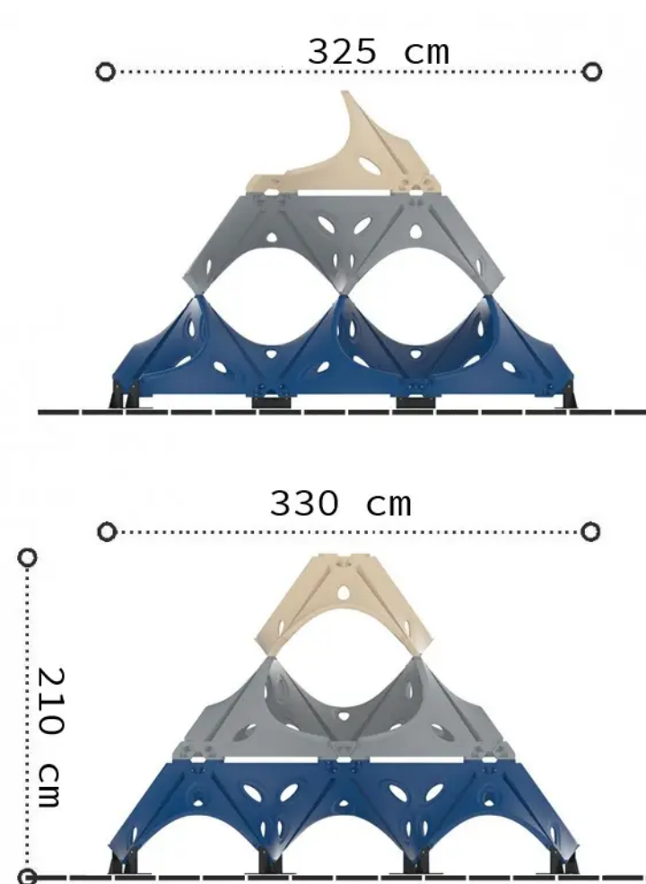
Rys. 1. Wymiary urządzenia
