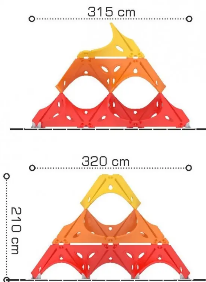
Rys. 1. Wymiary urządzenia
