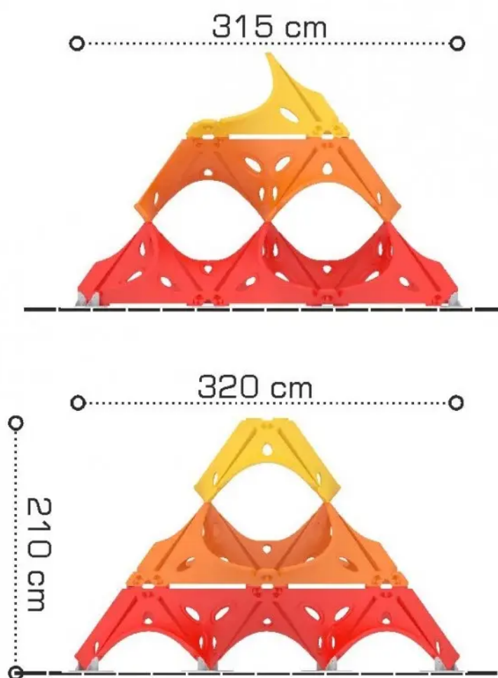
Rys. 1. Wymiary urządzenia
