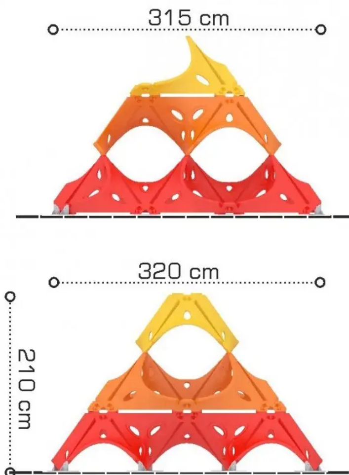
Rys. 1. Wymiary urządzenia
