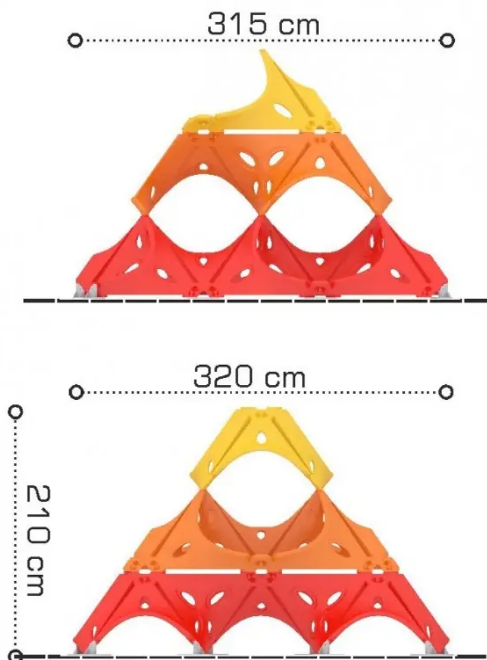
Rys. 1. Wymiary urządzenia
