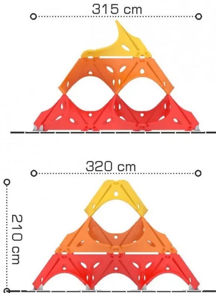
Rys. 1. Wymiary urządzenia
