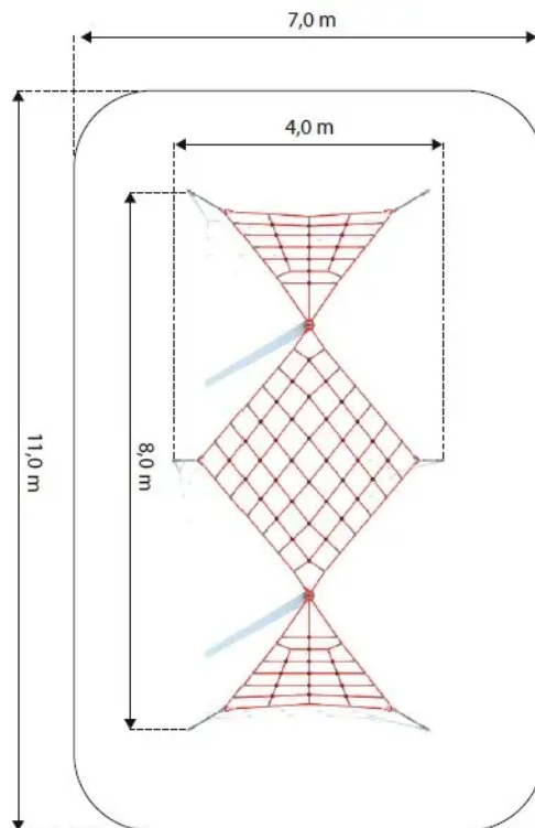
Rys. 1. Wymiary urządzenia i strefy bezpieczeństwa
