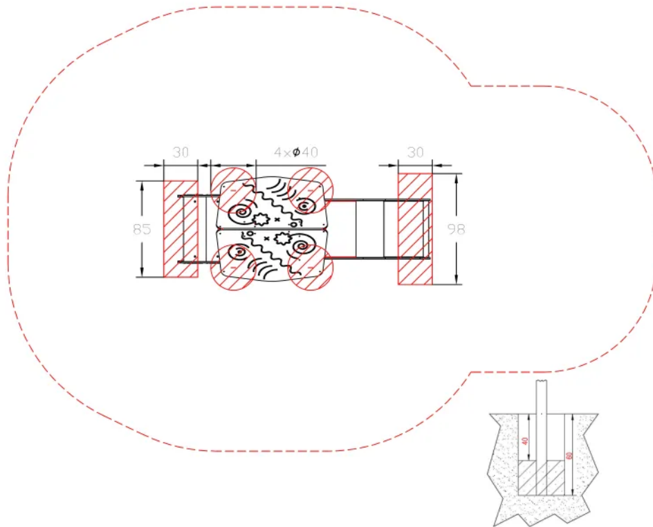
Rys. 2. Fundamenty
