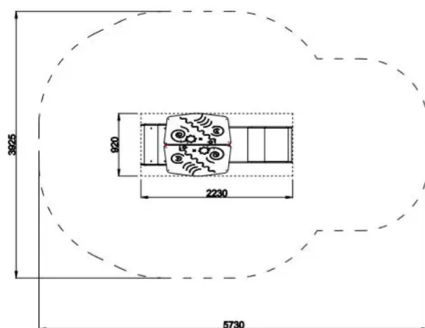
Rys. 1. Wymiary urządzenia i strefy bezpieczeństwa
