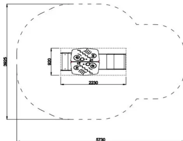
Rys. 1. Wymiary urządzenia i strefy bezpieczeństwa
