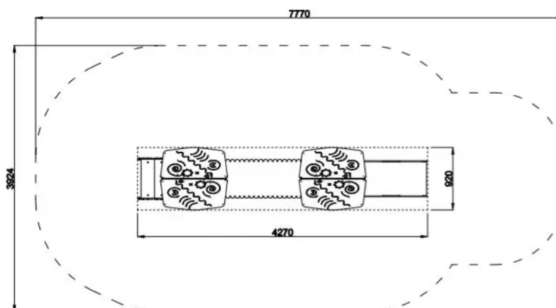
Rys. 1. Wymiary urządzenia i strefy bezpieczeństwa
