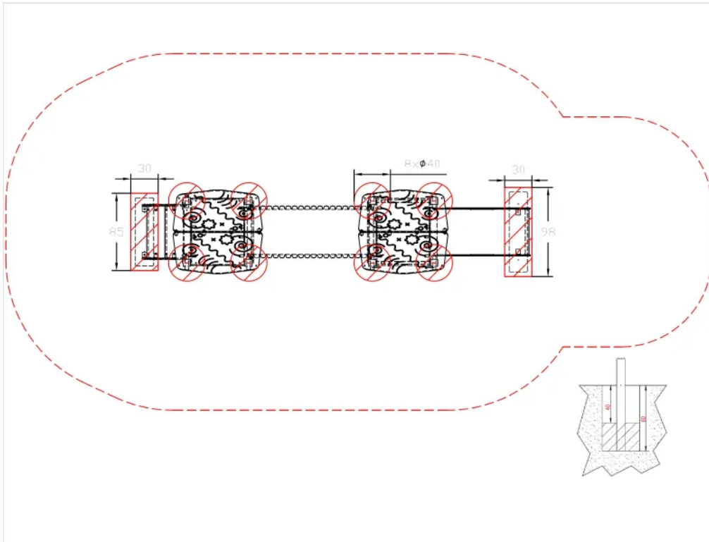
Rys. 2. Fundamenty
