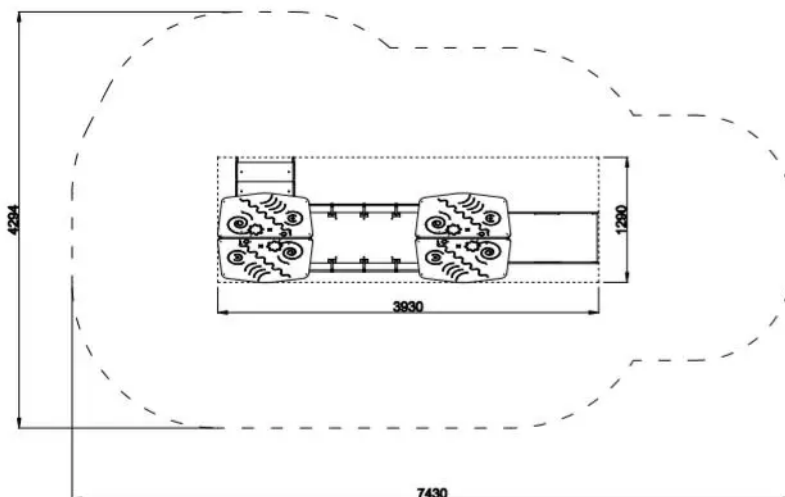
Rys. 1. Wymiary urządzenia i strefy bezpieczeństwa
