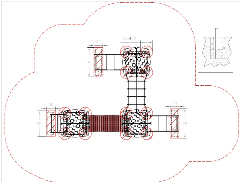
Rys. 2. Fundamenty
