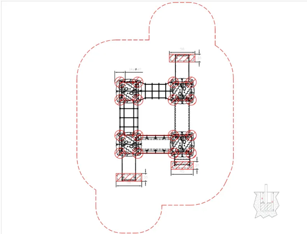
Rys. 2. Fundamenty
