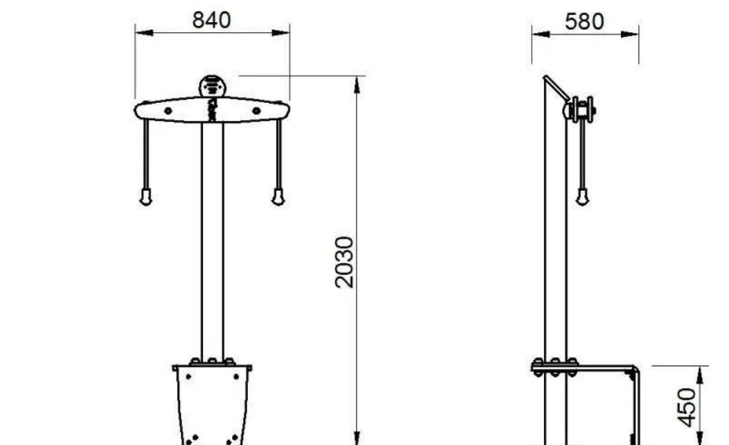
Rys. 1. Wymiary urządzenia
