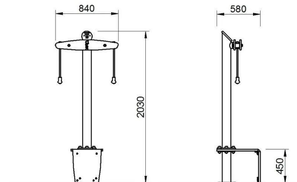
Rys. 1. Wymiary urządzenia
