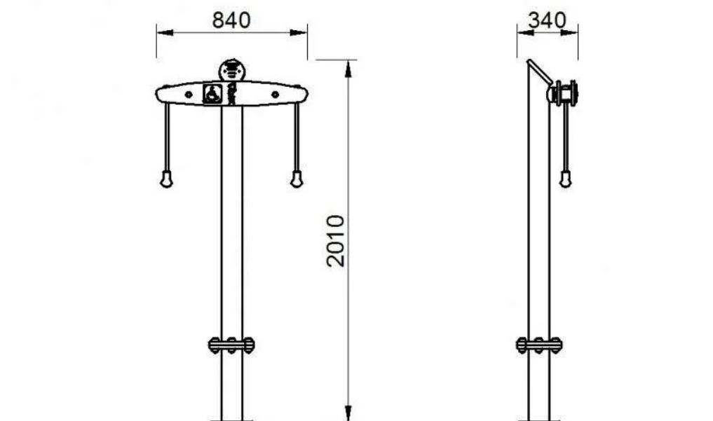
Rys. 1. Wymiary urządzenia
