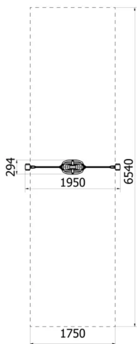
Rys. 1 Wymiary urządzenia i strefy bezpieczeństwa
