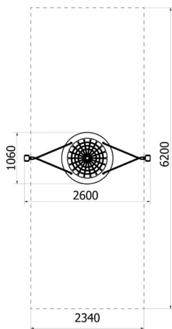
Rys. 1. Wymiary urządzenia
