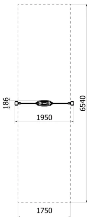
Rys. 1 Wymiary urządzenia i strefy bezpieczeństwa
