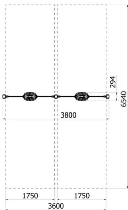
Rys. 1. Wymiary urządzenia i strefy bezpieczeństwa
