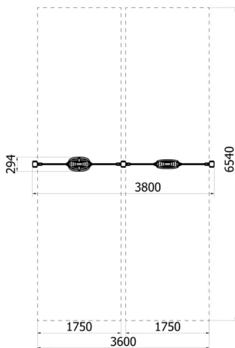
Rys. 1. Wymiary urządzenia i strefy bezpieczeństwa
