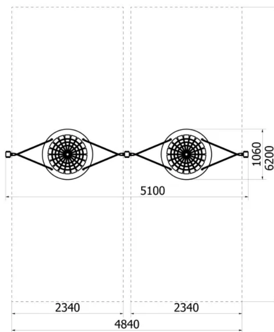
Rys. 1. Wymiary urządzenia i strefy bezpieczeństwa
