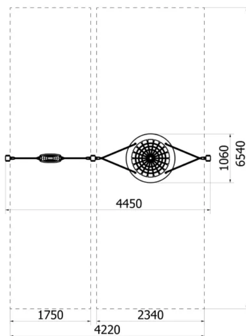
Rys. 1. Wymiary urządzenia i strefy bezpieczeństwa
