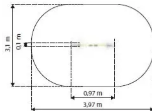
Rys. 1. Wymiary urządzenia i strefy bezpieczeństwa
