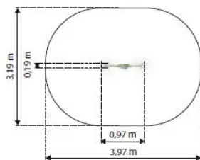
Rys. 1. Wymiary urządzenia i strefy bezpieczeństwa
