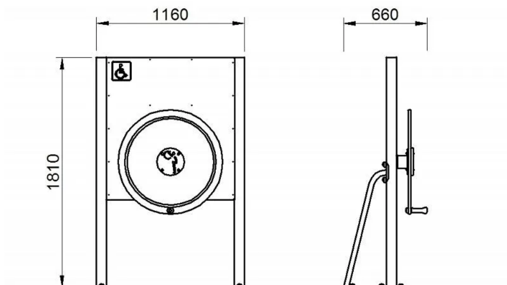
Rys. 1. Wymiary urządzenia
