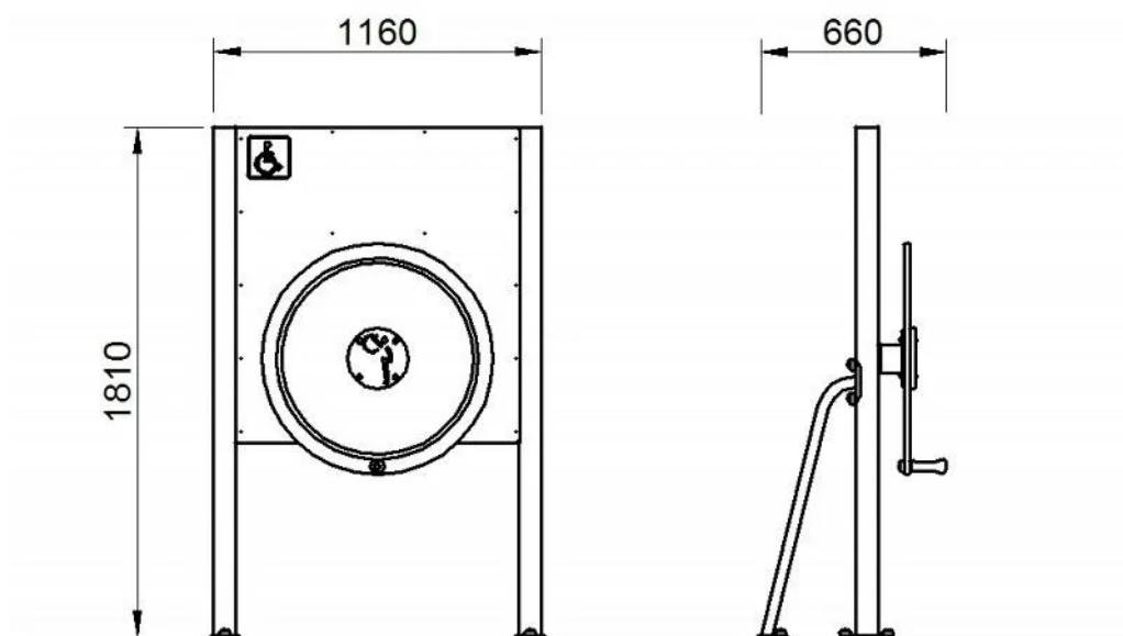
Rys. 1. Wymiary urządzenia
