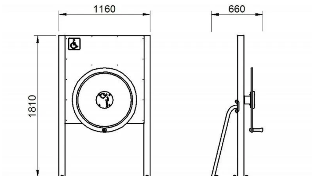
Rys. 1. Wymiary urządzenia
