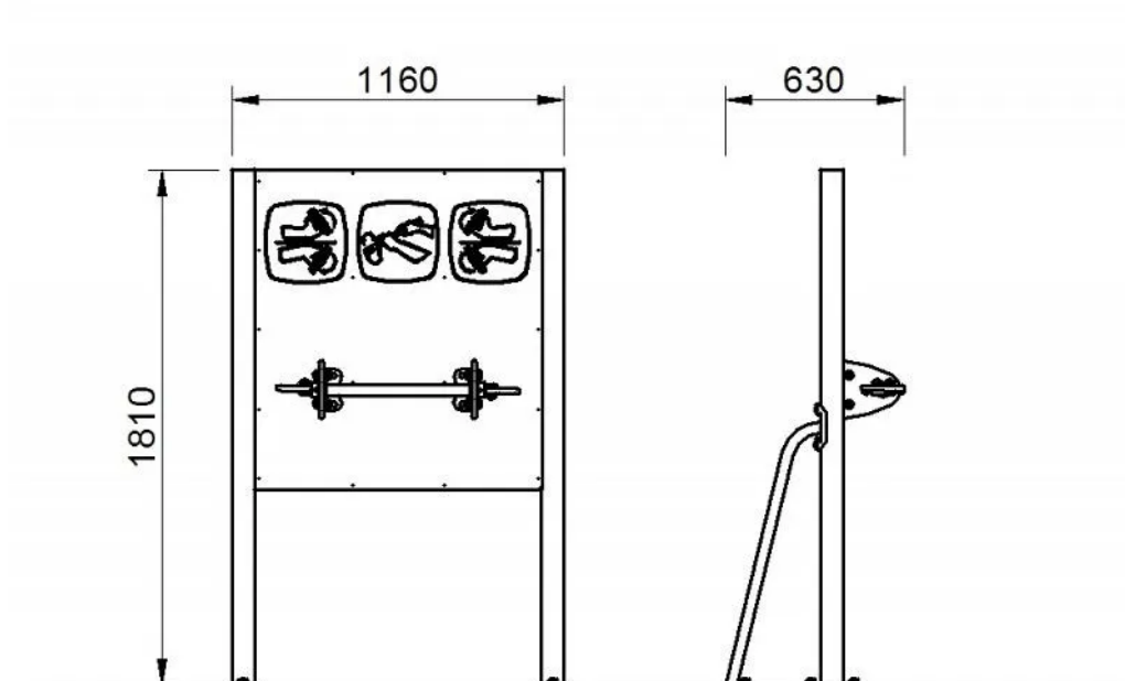
Rys. 1. Wymiary urządzenia
