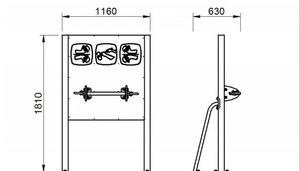
Rys. 1. Wymiary urządzenia
