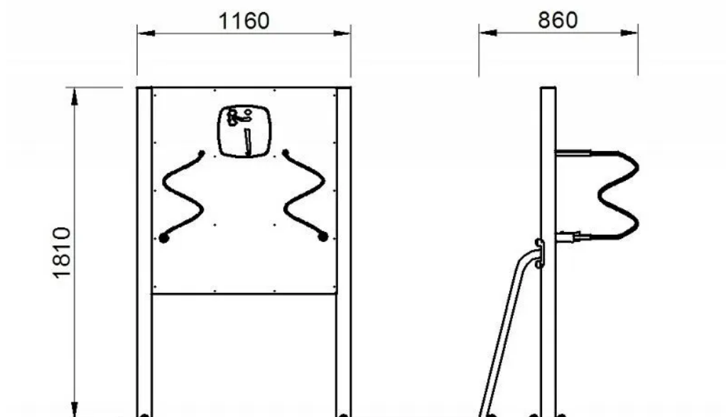
Rys. 1. Wymiary urządzenia
