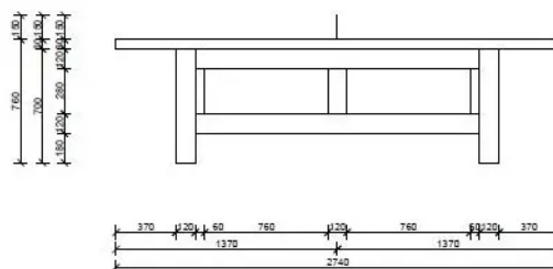
Rys. 1. Wymiary urządzenia
