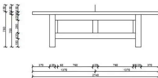
Rys. 1. Wymiary urządzenia
