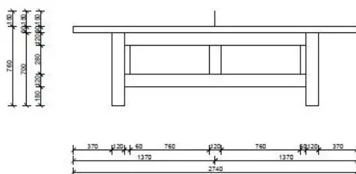
Rys. 1. Wymiary urządzenia
