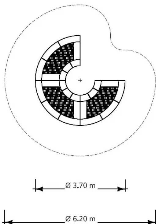
Rys. 1. Wymiary urządzenia i strefy bezpieczeństwa
