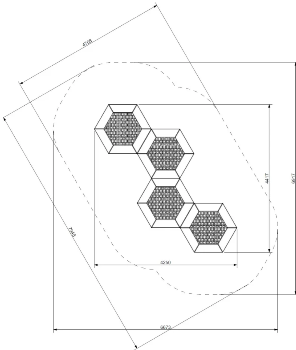
Rys. 1. Wymiary urządzenia i strefy bezpieczeństwa
