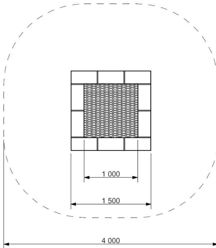
Rys. 1. Wymiary urządzenia i strefy bezpieczeństwa
