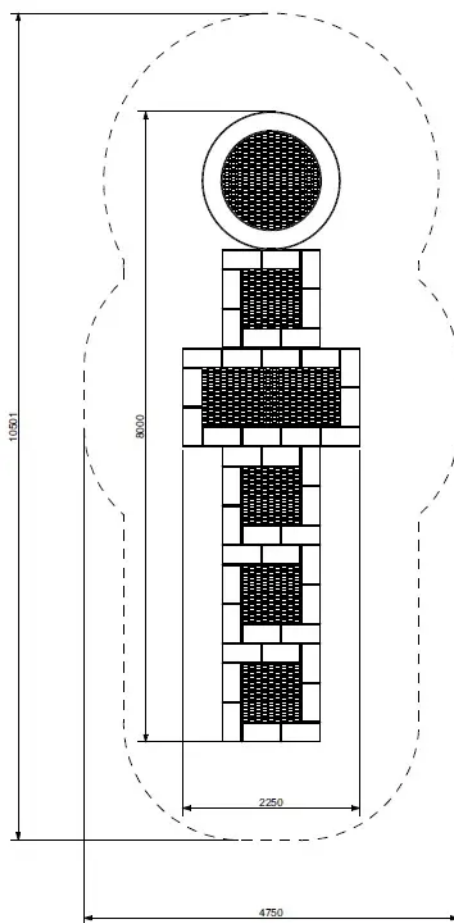
Rys. 1. Wymiary urządzenia i strefy bezpieczeństwa
