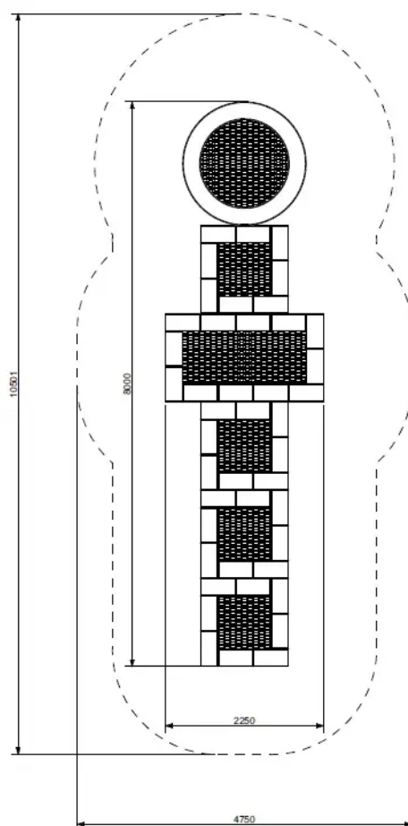
Rys. 1. Wymiary urządzenia i strefy bezpieczeństwa
