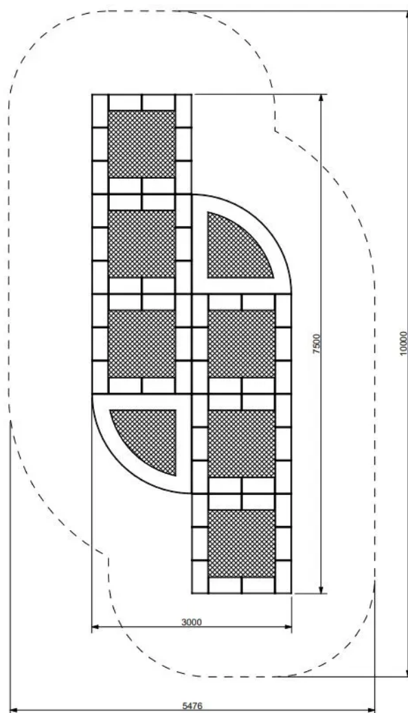
Rys. 1. Wymiary urządzenia i strefy bezpieczeństwa
