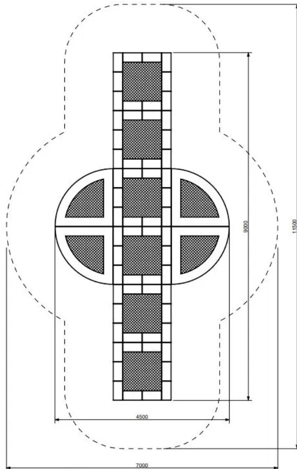
Rys. 1. Wymiary urządzenia i strefy bezpieczeństwa
