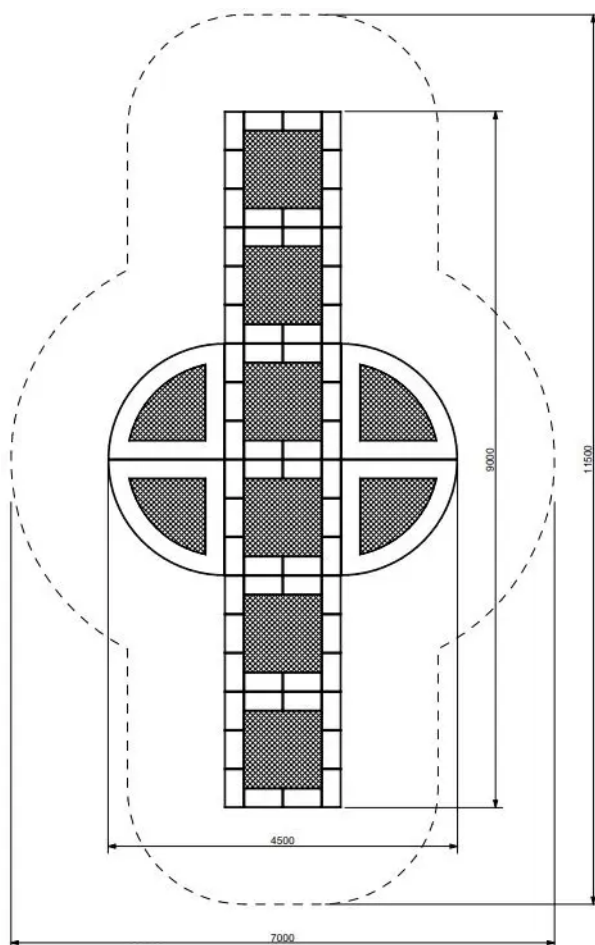
Rys. 1. Wymiary urządzenia i strefy bezpieczeństwa
