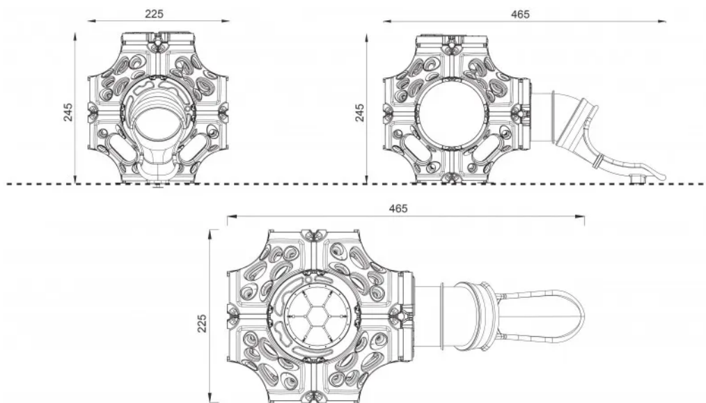
Rys. 1. Wymiary urządzenia
