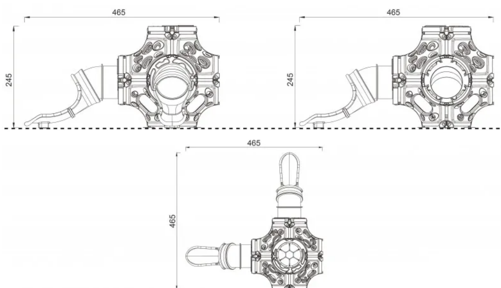
Rys. 1. Wymiary urządzenia
