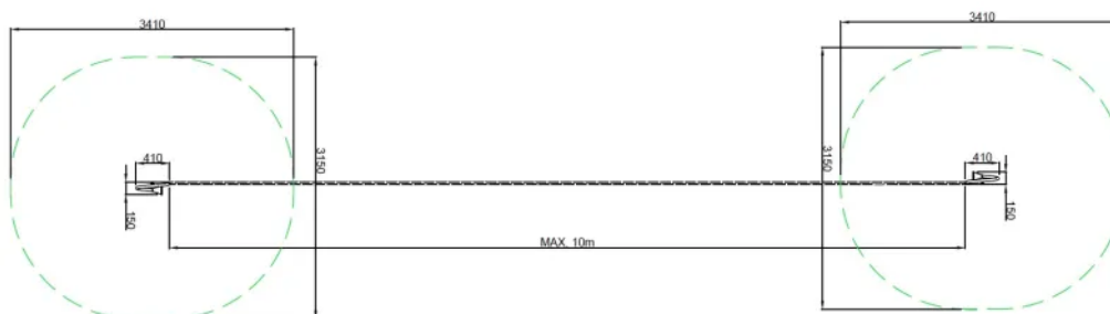
Rys. 1. Wymiary urządzenia i strefy bezpieczeństwa
