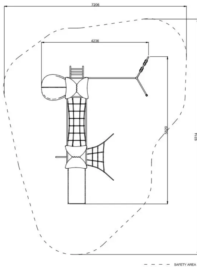
Rys. 1. Wymiary urządzenia i strefy bezpieczeństwa
