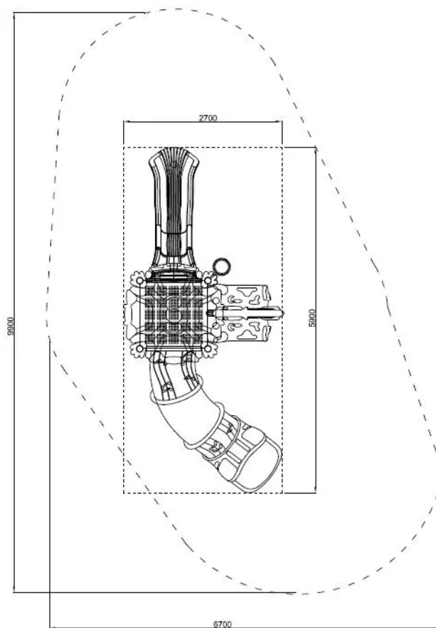
Rys. 1. Wymiary urządzenia i strefy bezpieczeństwa
